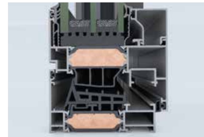
ELVIAL I 2 _ ΚΑΙΝΟΤΟΜΟΣ ΤΕΧΝΟΛΟΓΙΑ ΜΟΝΩΣΗΣ ΑΦΡΩΔΕΣ ΚΕΝΤΡΙΚΟ ΕΛΑΣΤΙΚΟ ΔΙΠΛΗΣ ΔΙΕΛΑΣΗΣ ΑΦΡΩΔΕΣ ΘΕΡΜΟΜΟΝΩΤΙΚΟ ΠΡΟΦΙΛ
