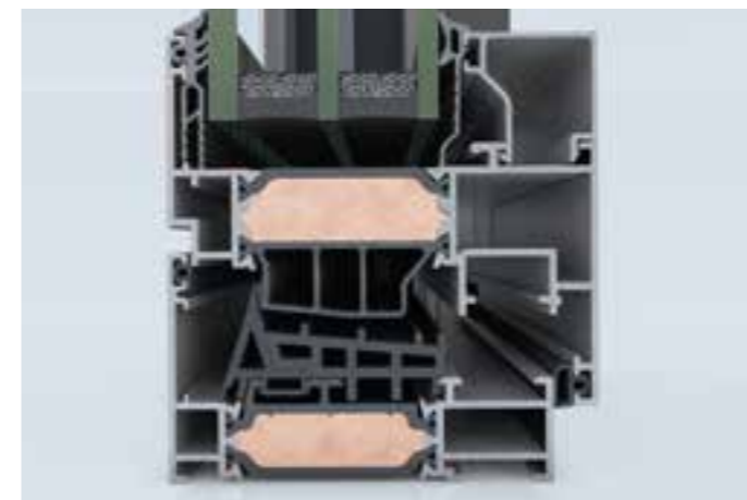
ELVIAL I 2 _ ΚΑΙΝΟΤΟΜΟΣ ΤΕΧΝΟΛΟΓΙΑ ΜΟΝΩΣΗΣ ΑΦΡΩΔΕΣ ΚΕΝΤΡΙΚΟ ΕΛΑΣΤΙΚΟ ΔΙΠΛΗΣ ΔΙΕΛΑΣΗΣ
